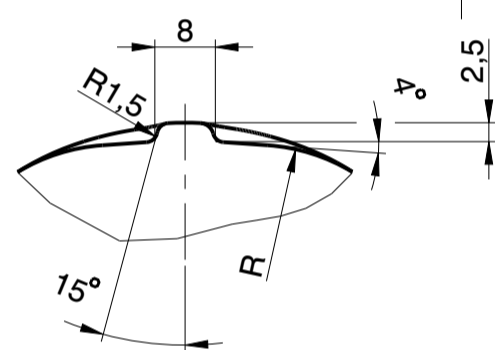
Schnitt A-A
