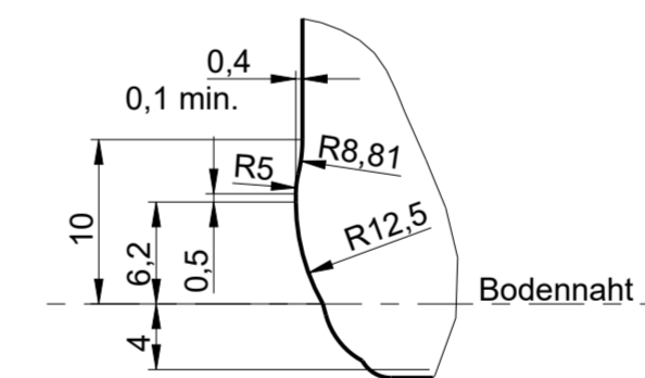
DETAIL ETIKETTENSCHUTZ SCHNITT A-A 2:1
