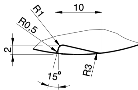
Schnitt B-B 2:1
