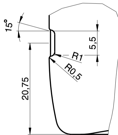
Schnitt A-A 2:1
