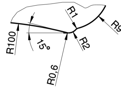
Detail A 2:1
