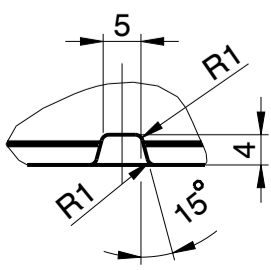
Detail: Bodennocke
