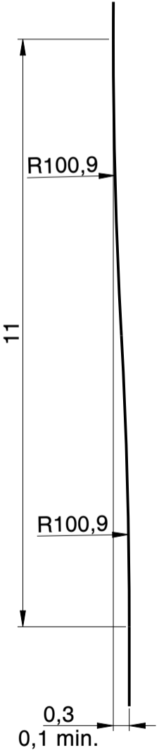
Detail "Y" M.: 10:1
