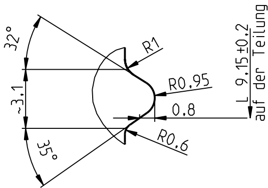
Detail Gewinde 5:1
